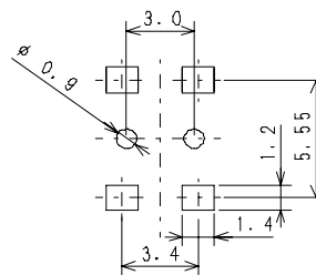
基板パターン参考図 5/1 Copper pattern example for P.C.B
